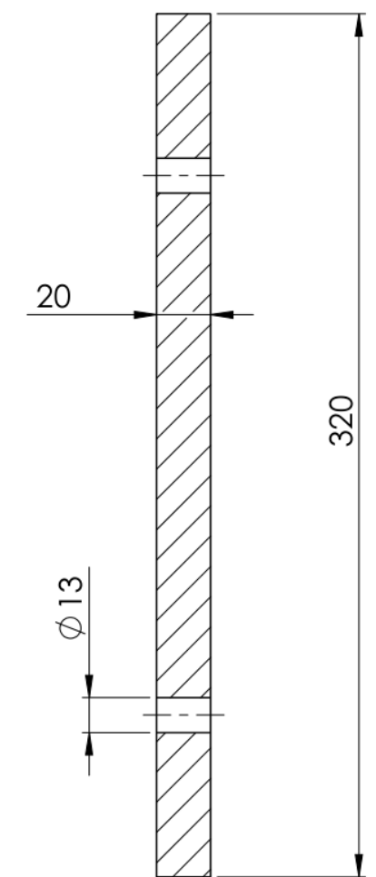
SCHNITT B-B
