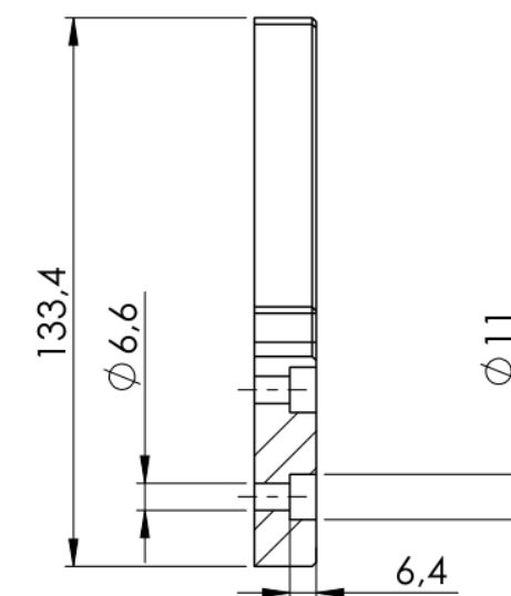
SCHNITT A-A
