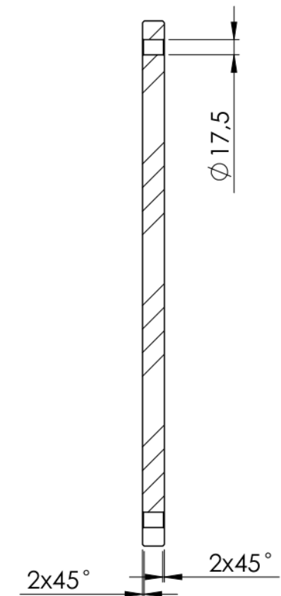
SCHNITT A-A
