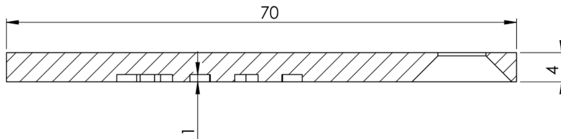
SCHNITT B-B
