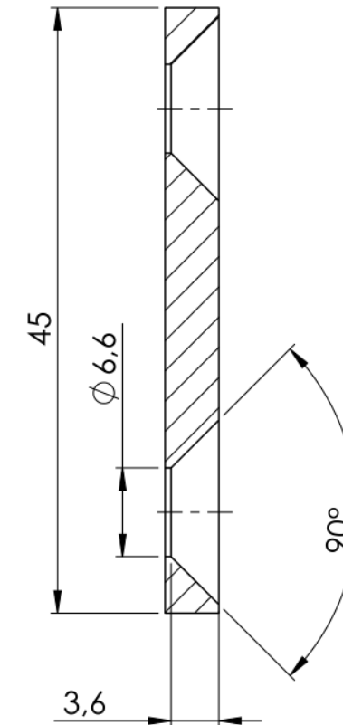
SCHNITT A-A
