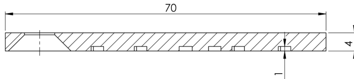
SCHNITT B-B
