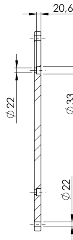
SCHNITT A-A
