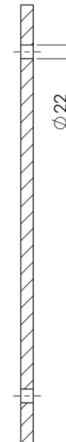
SCHNITT A-A MAßSTAB 1 : 6
