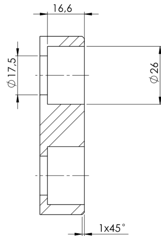
SCHNITT A-A
