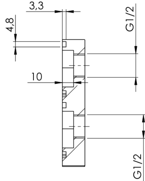
SCHNITT A-A MAßSTAB 1 : 2
