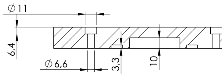
SCHNITT B-B MAßSTAB 1 : 2
