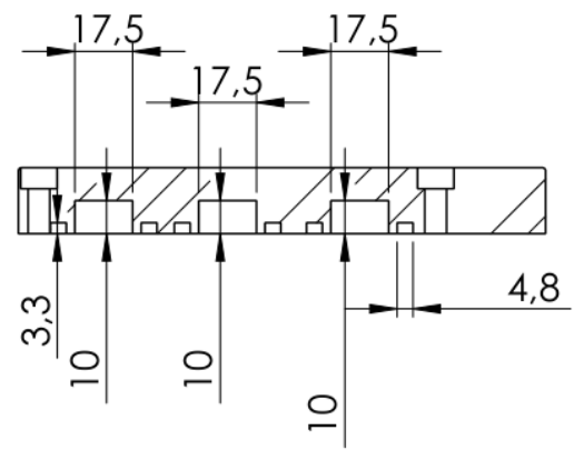
SCHNITT A-A MAßSTAB 1 : 2.5
