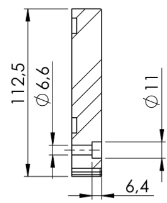
SCHNITT B-B MAßSTAB 1 : 2.5
