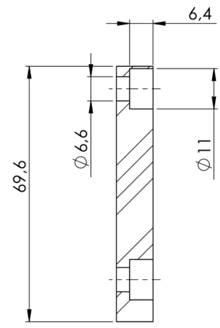
SCHNITT A-A
