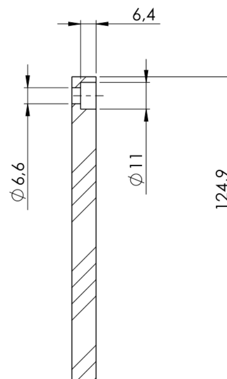
SCHNITT A-A MAßSTAB 1 : 1.5
