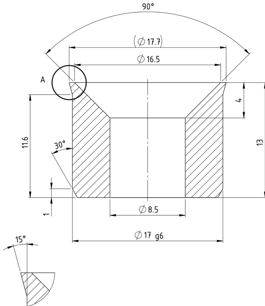
DETAIL A 10 : 1
