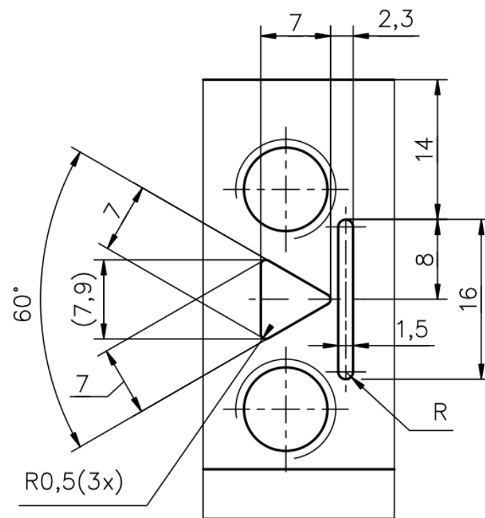
B (2 : 1)
