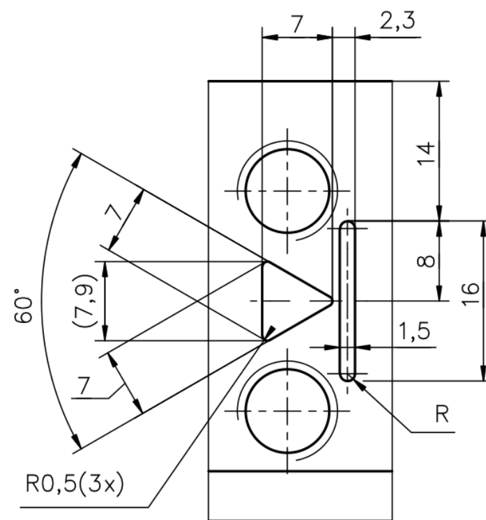
B (2 : 1)
