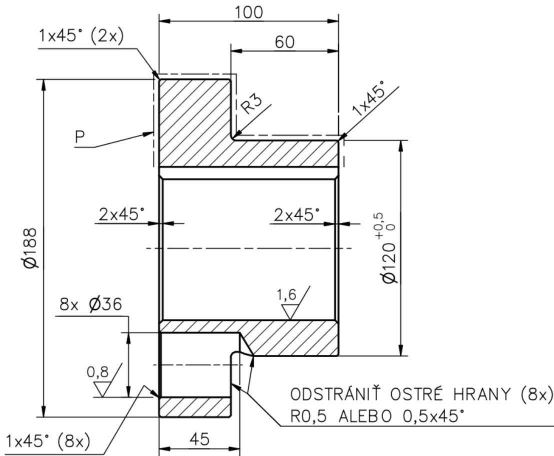
A-A (1 : 2)
