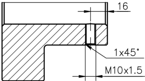
B-B (1 : 2)
