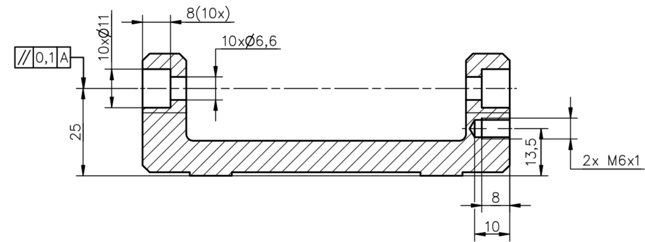
B-B (1 : 1)
