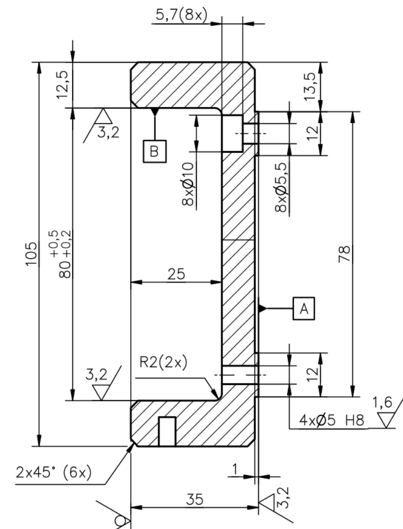
A-A (1 : 1)
