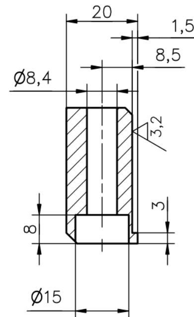
A-A (1 : 1)
