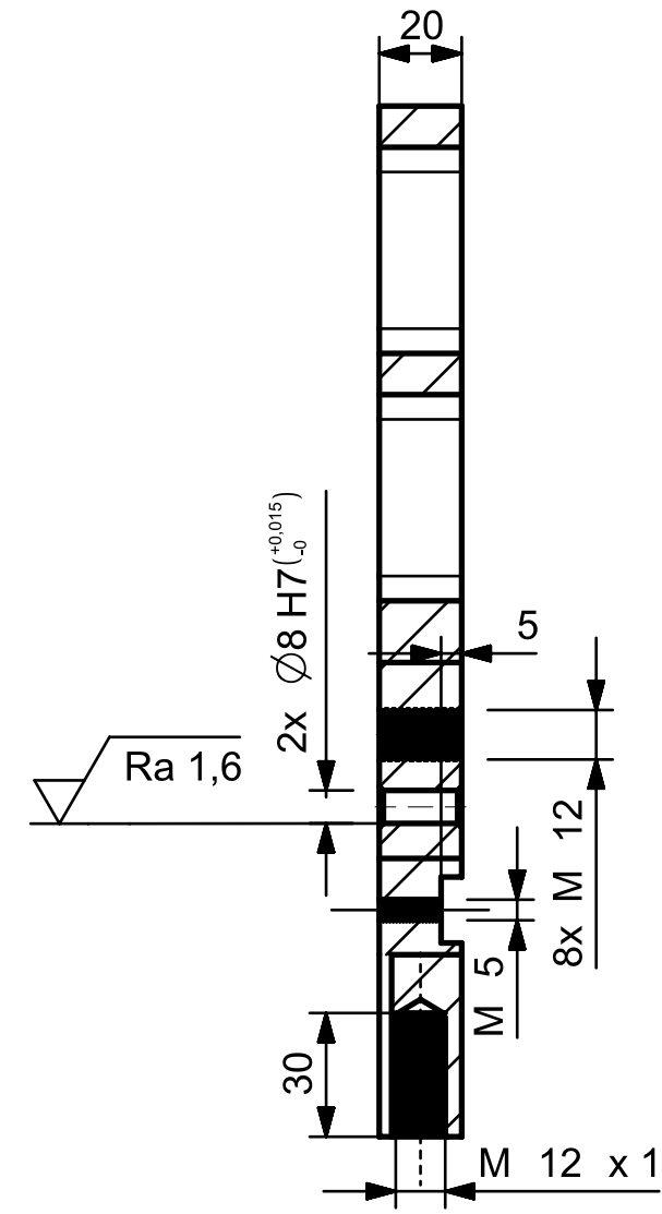
SECTION A-A
