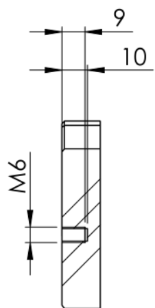
SCHNITT B-B
