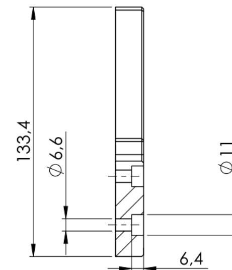
SCHNITT A-A
