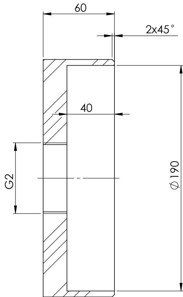
SCHNITT A-A
