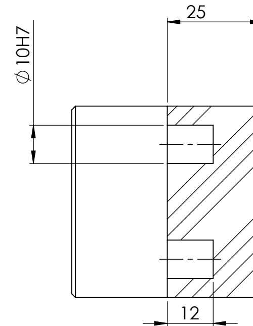
SCHNITT B-B
