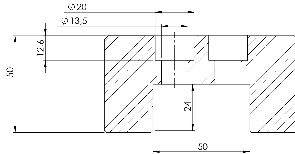
SCHNITT A-A
