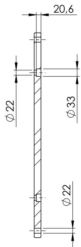
SCHNITT A-A
