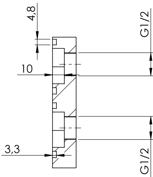
SCHNITT A-A MAßSTAB 1 : 2
