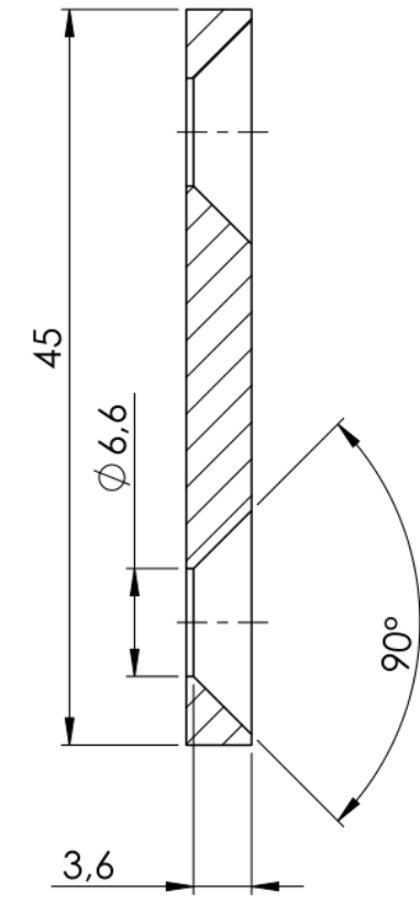
SCHNITT A-A
