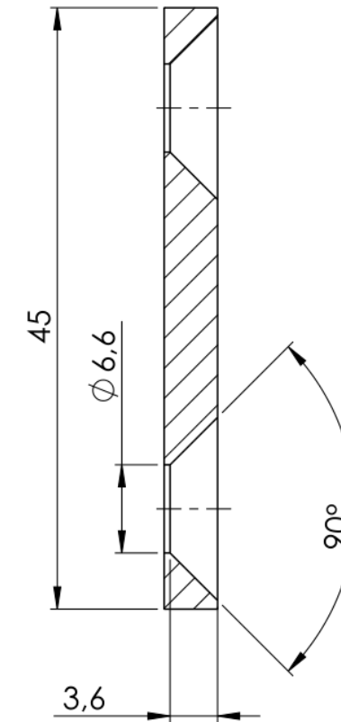
SCHNITT A-A
