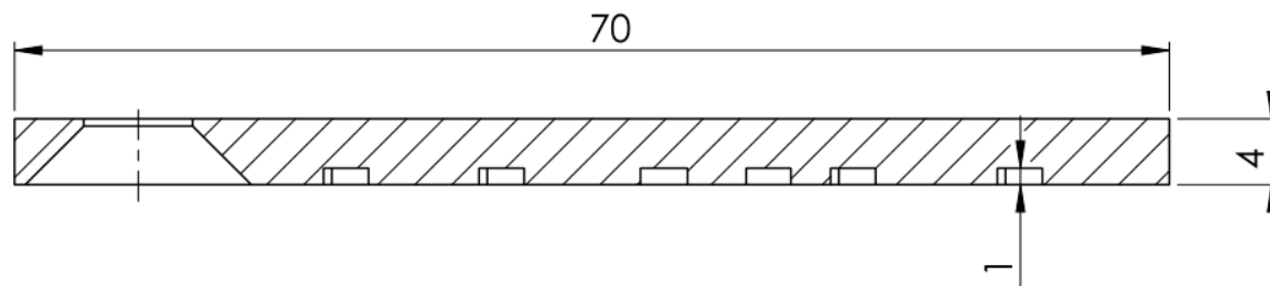
SCHNITT B-B
