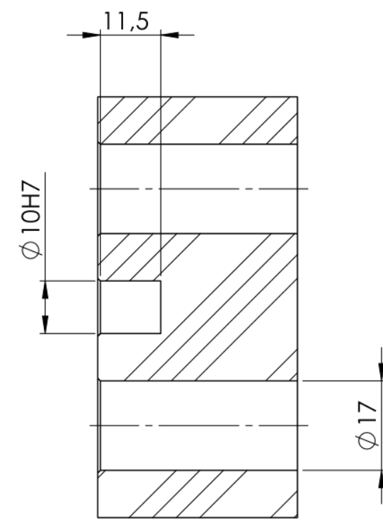
SCHNITT A-A
