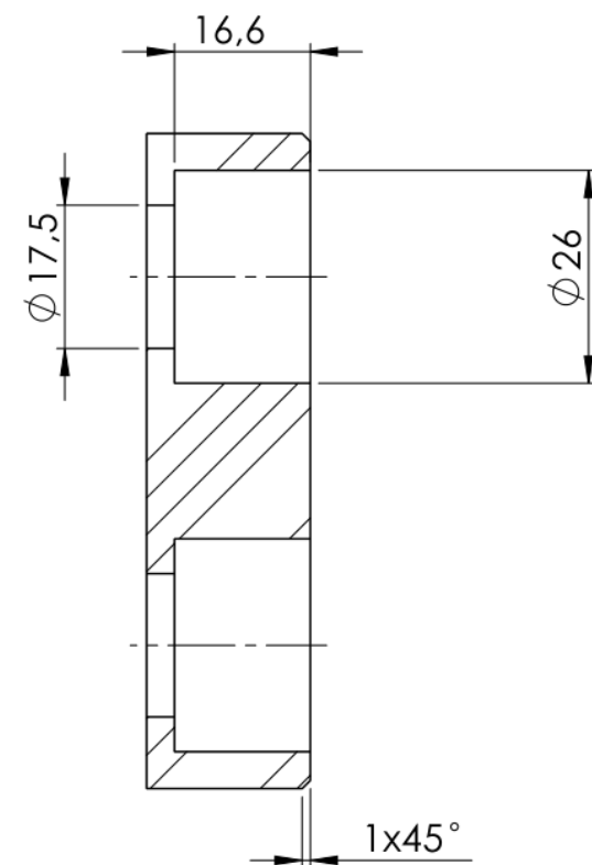
SCHNITT A-A
