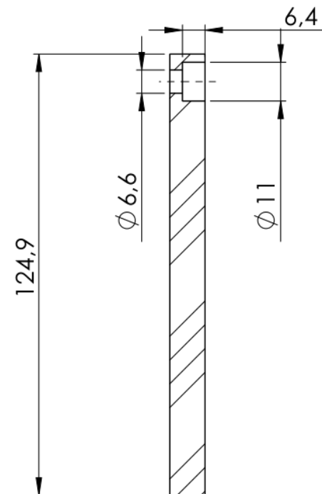
SCHNITT A-A MABSTAB 1 : 1.5
