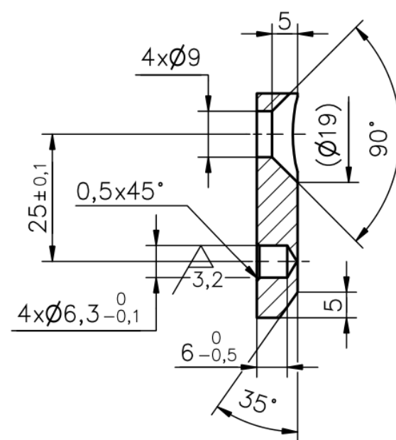
A-A (1 : 1)
