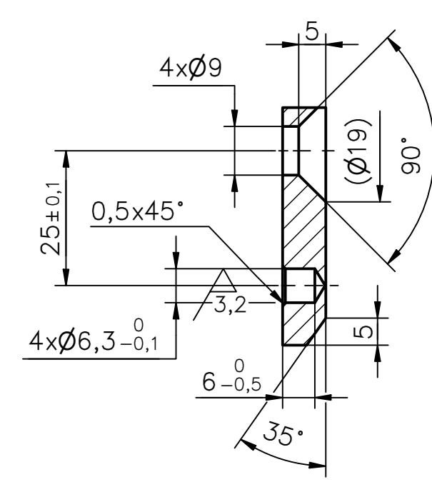
A-A (1 : 1)
