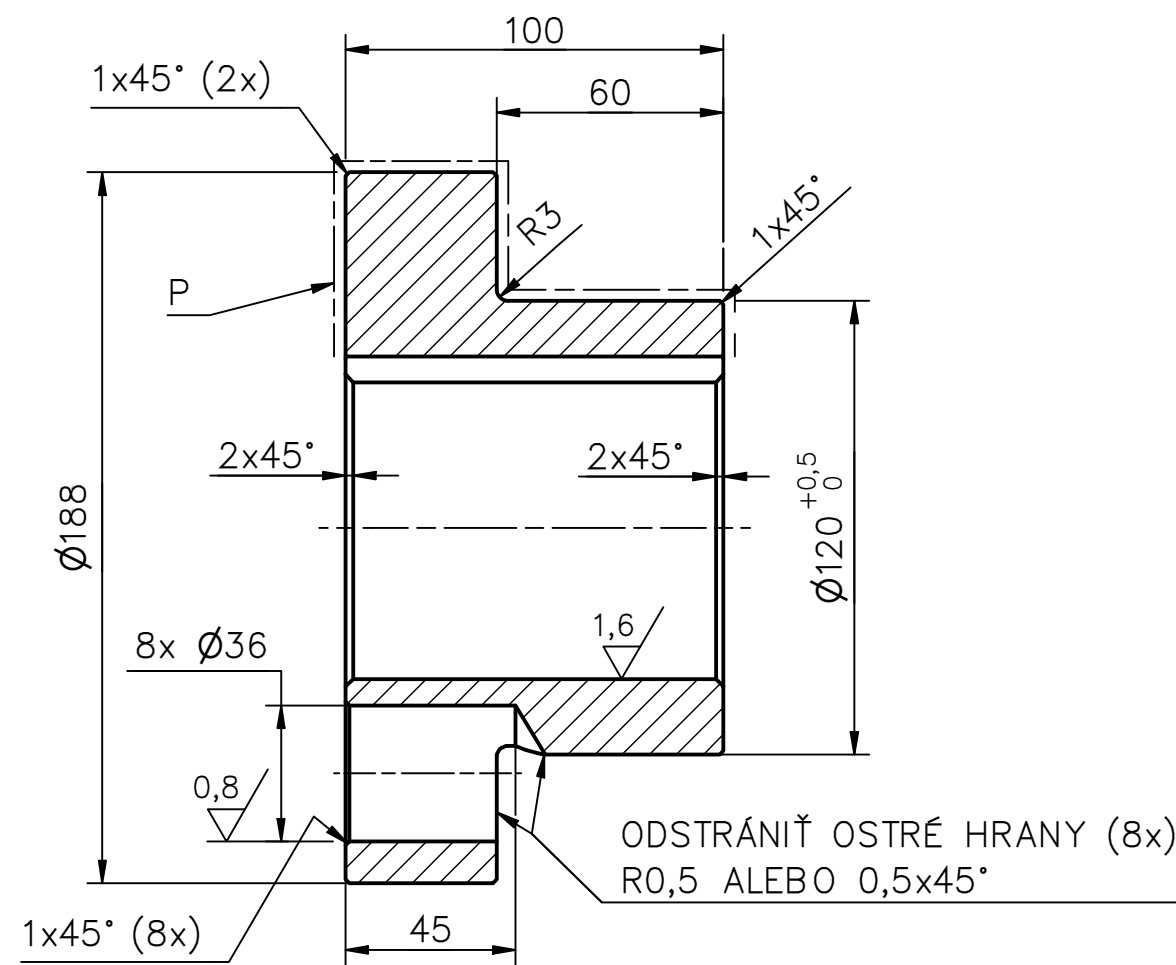
A-A (1 : 2)
