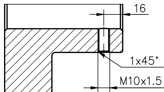
B-B (1 : 2)
