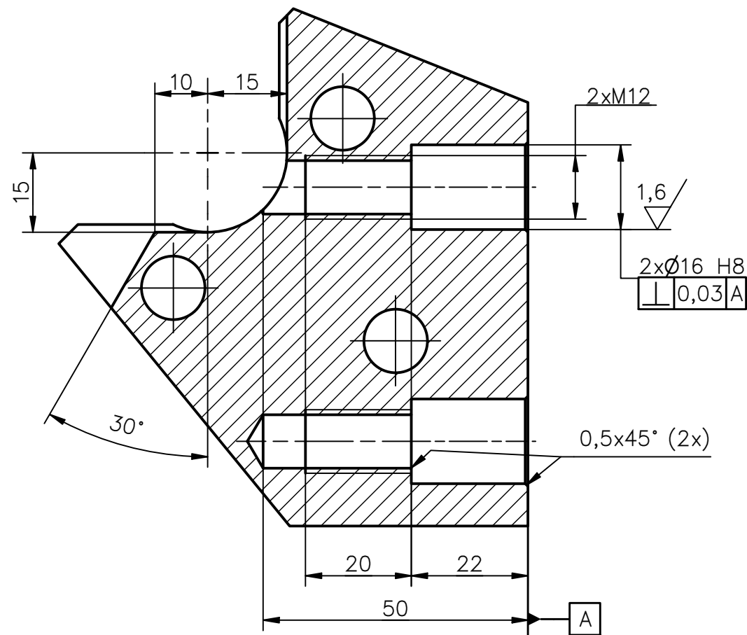
A-A (1 : 1)
