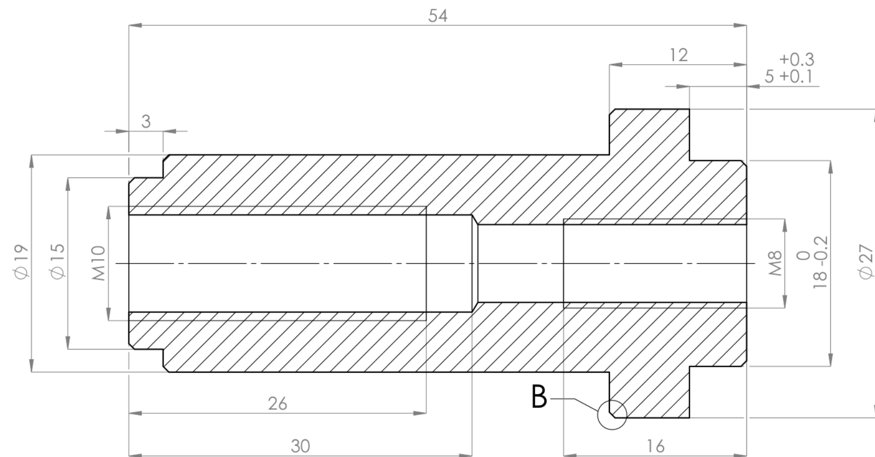
SECTION A-A
